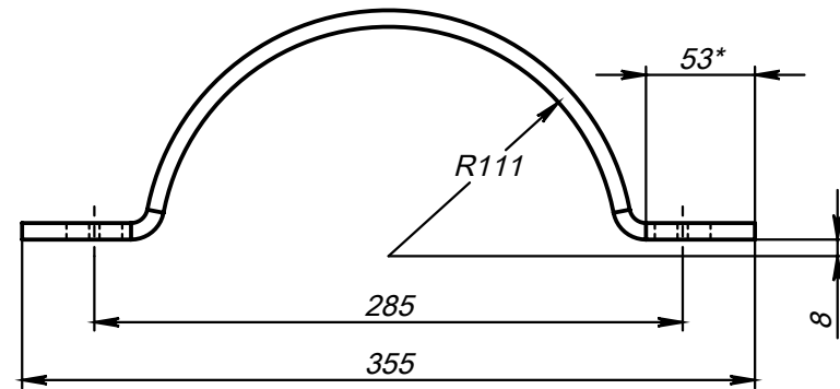
Поз.1 (Полухомут)
