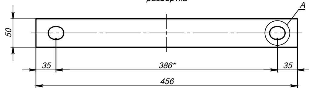
Поз.1 (Полухомут) развертка
